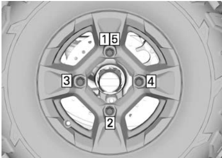
ANZUGSREIHENFOLGE
