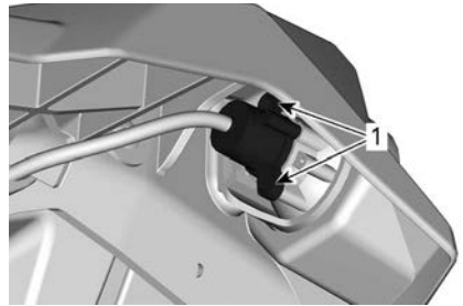
1. Borgschroef lens
