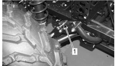
1. Borgpen van stabilisatiestang vergrendeld
