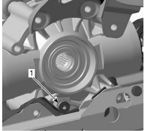
TRANSMISIÓN INTERMEDIA, PARTE IZQUIERDA DEL VEHÍCULO
