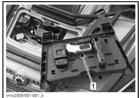
COMPARTIMENT D'ENTRETIEN AVANT 1. Télécommande de treuil
