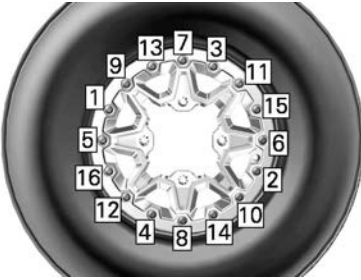
TYPISCH - AANDRAAIVOLGORDE
