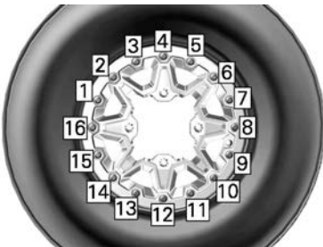
TIPIQUE - SÉQUENCE DE SERRAGE FINAL
