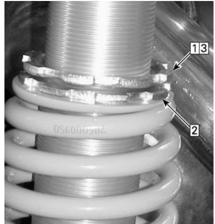
TYPIQUE – AMORTISSEUR AVEC RÉGLAGE FILETÉ
