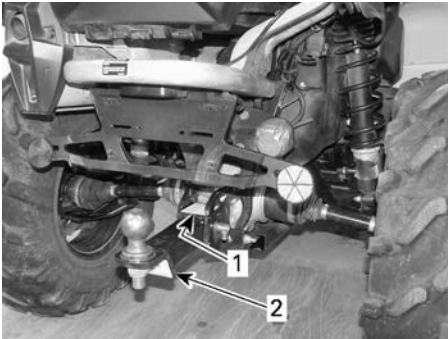
1. Anhängerkupplung 2. Sicherheitshinweisschild
