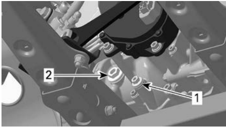
1. Ablaufstopfen 2. Ölstandskontrollschraube
