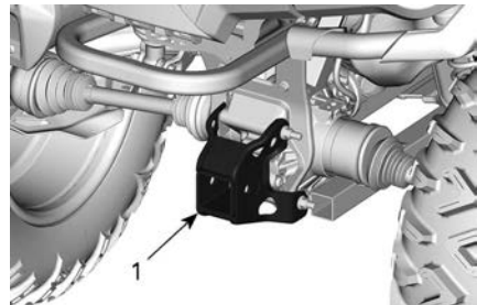
1. Perävaunun vetokoukku
