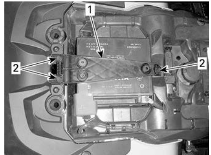
1. Batterie-Halteriemen 2. Halteschrauben
