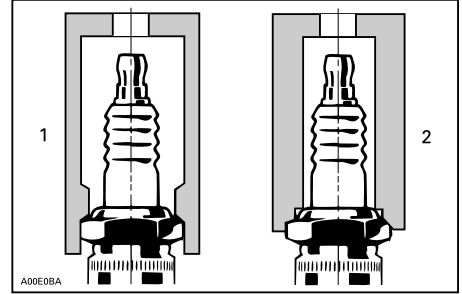
1. Hyväksytyt hylsyavain
