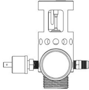
ACTIONNEUR CHARGÉ
