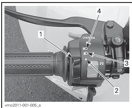
TÍPICA — FUNÇÕES DO INTERRUPTOR DOS FARÓIS DIANTEIROS
