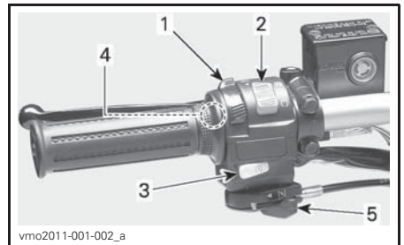
TÍPICA — INTERRUPTOR MULTIFUNCIONAL
