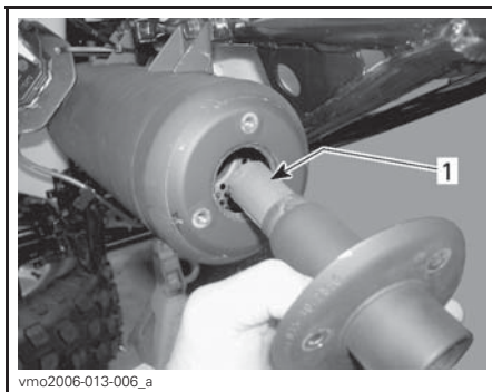
TYPISCH 1. Funkenschutz
