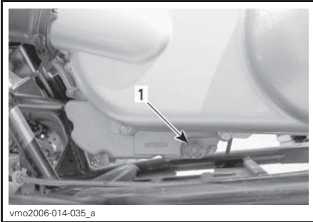
LINKS UNTER DER CVT-ABDECKUNG
