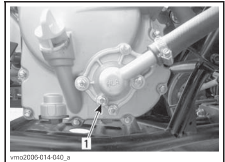
1. Kühlsystemablassschraube
