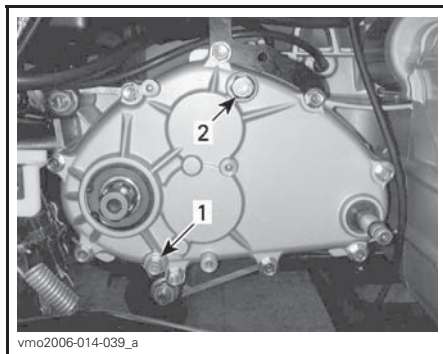
1. Getriebe-Ablassschraube 2. Getriebe-Einfüllschraube
