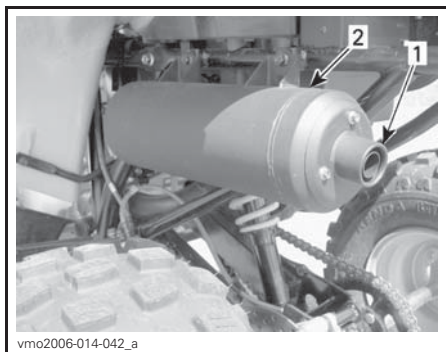
TYPISCH 1. Ausgang des Auspufftopfs entfernen 2. Auspuff
