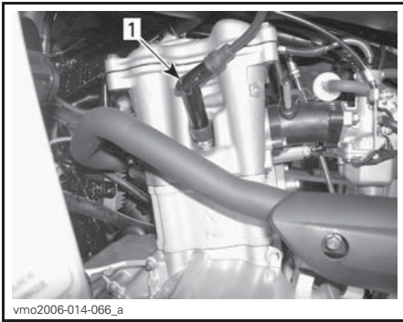
vmz2006-014-066_a LINKE MOTORSEITE 1. Zündkerze
