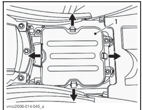
1. Deckel des Luftfilterkastens
