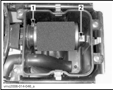
TYPIQUE - VAPORISER DU NETTOYEUR DE CHAQUE CÔTÉ DE L'ÉLÉMENT
