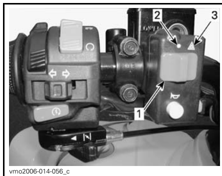
1. Interrupteur des feux de détresse 2. Position «OFF» 3. Position «DÉTRESSE»
