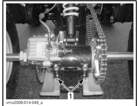
TYPIQUE 1. Boulons de blocage du tendeur de chaîne
