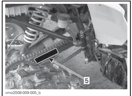
5. Ubicación de la etiqueta de ajuste de la cadena de transmisión
