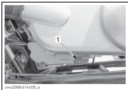
PARTE IZQUIERDA, DEBAJO DE LA CUBIERTA DE LA TRANSMISIÓN CVT 1. Tapón de drenaje de aceite
