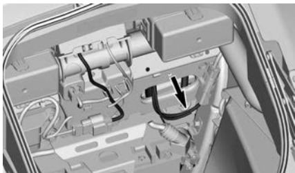
DC12 - 前客户配件电路 - 储物舱后方
