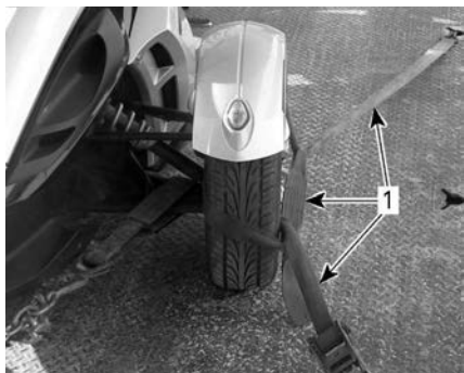
前轮固定 - 典型示例方法 2
