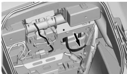
DC12 - CIRCUITO ACCESSORIO DEL CLIENTE ANTERIORE - DIETRO LO SCOMPARTO ANTERIORE
