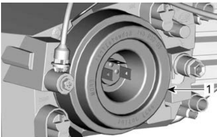
1. Cappuccio dell'alloggiamento
