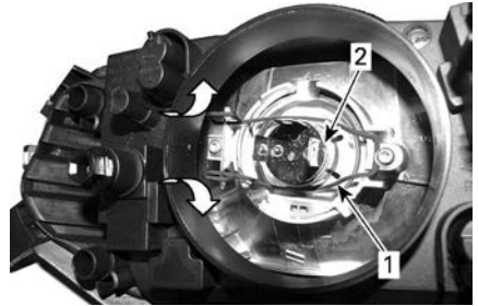
1. Molla che fissa la lampadina 2. Alloggiamento lampadina
