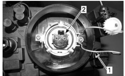
1. Molla che fissa la lampadina 2. Alloggiamento lampadina
