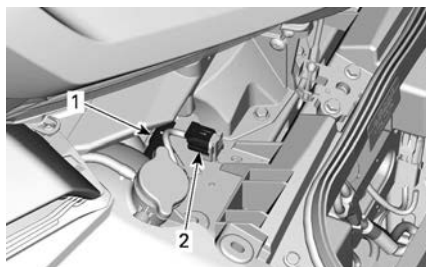
1. Connettore diagnostico (per BUDS2) 2. Connettore OBD2 a 6 pin
