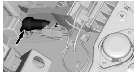
DC56 – HINTERER ZUBEHÖRSCHALT-KREIS DES KUNDEN – UNTER DEM BEIFAHRERSITZ
