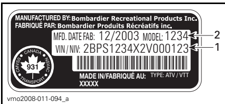
1. NIV (Numéro d'Identification du Véhicule) 2. Modèle
