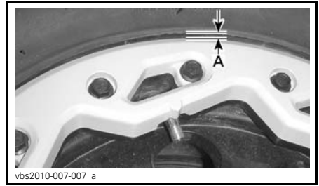
A. Jeu égal tout autour de l'anneau de retenue du verrou de talon
