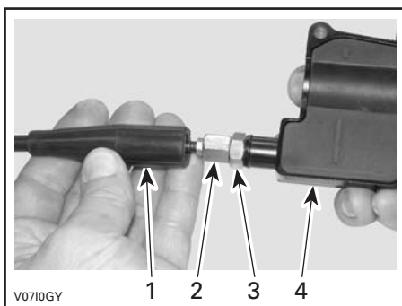
1. Protecteur de câble 2. Tendeur de câble d'accélérateur 3. Écrou de blocage 4. Logement de la manette d'accélérateur
