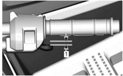
1. 2 mm. 079 Zoll
