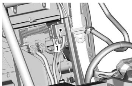
1. Bakre säkringsdosa
