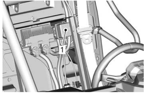
1. Bakre sikringsboks
