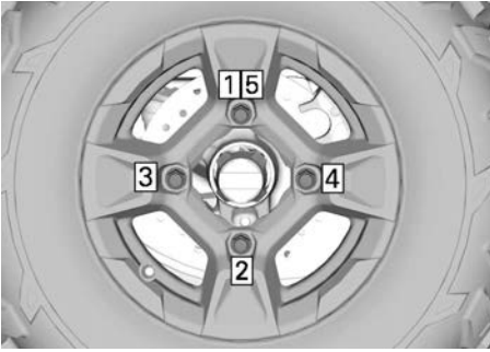
STRAMMEREKKEFØLGE
