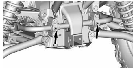
TYPISK – BAKRE STABILISATORSTAG
