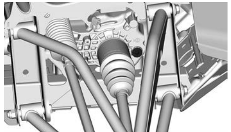
AVEC ACTIONNEUR 4RM INTÉGRÉ
