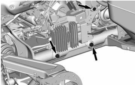
TORNILLOS DEL SOPORTE DEL REGULADOR/VOLTAJE
