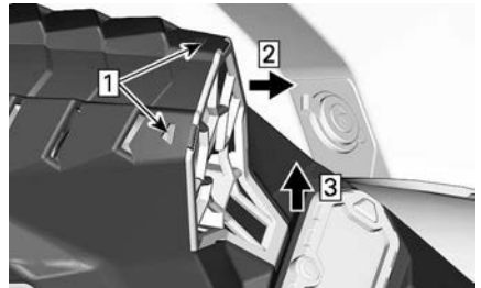
1. Filtro dell'aria CVT
