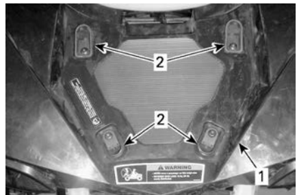
1. Ladefläche 2. Kunststoffösen
