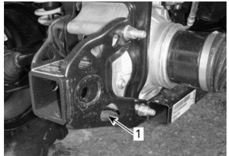
1. Hinterer Verzurrpunkt
