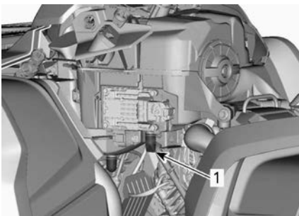
1. Luftfiltergehäuse-Einlass-Ablassrohr
