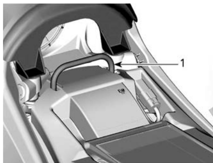
1. Удерживающая скоба
