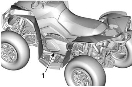
1. Крышка вариатора
