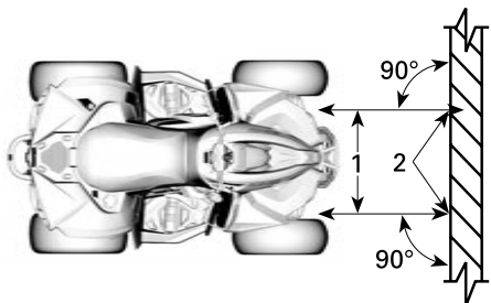
1. Центральные линии для регулировки фар головного освещения
