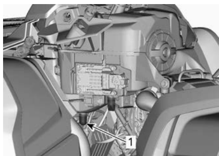
1. Дренажная трубка корпуса воздушного фильтра.
