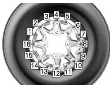
代表例 - 最後の締め付け順序
