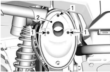
1. Limpieza del supresor de chispas
