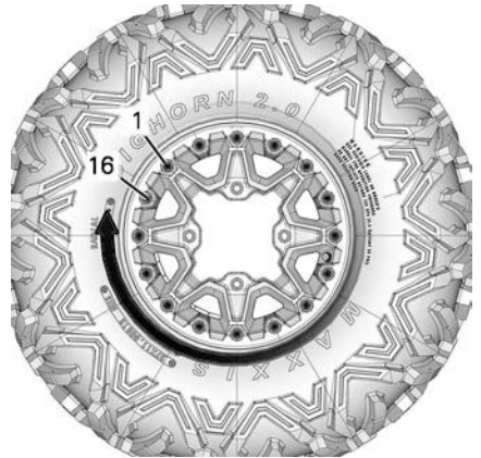
TÍPICO: SECUENCIA DE APRIETE FINAL
