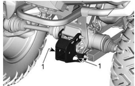
1. Abschlepphaken
