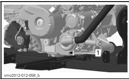
vmo2012-012-058_b 1. Kühlmittelablassschraube
