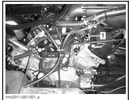
tmo2011-001-501_a 1. Entlüftungsschraube des vorderen Zylinders
