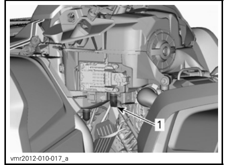
TYPISCH - EINIGE TEILE AUS GRÜNDEN DER ÜBERSICHTLICHKEIT ENTFERNT 1. Luftfiltergehäuse-Einlass-Ablassrohr
