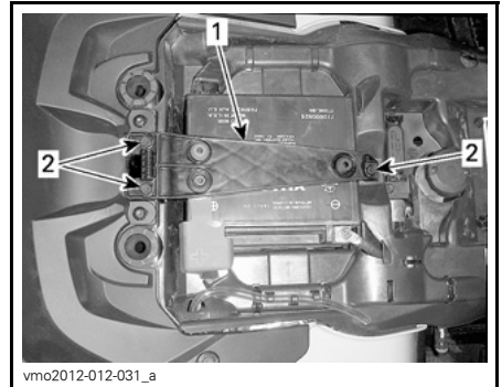
1. Batteriehalteriem 2. Halteschrauben
