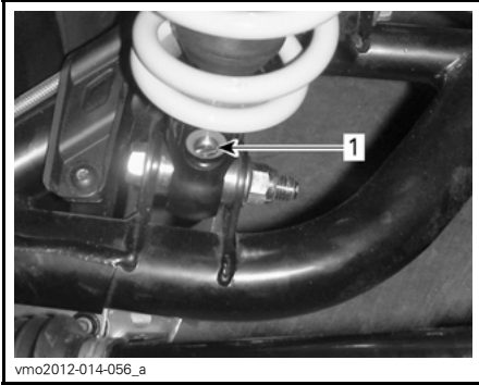
1. Rückstoßregler (Schraubendreher erforderlich)
