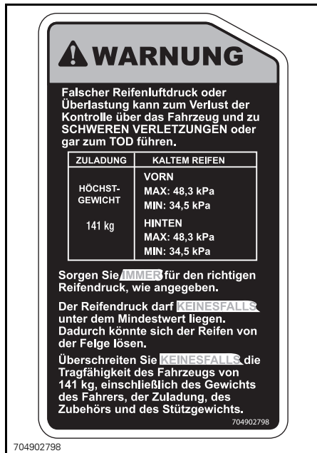
HINWEISSCHILD 6 (ZUTREFFENDE WERTE ENTNEHMEN SIE DEN TECHNISCHEN DATEN.)
