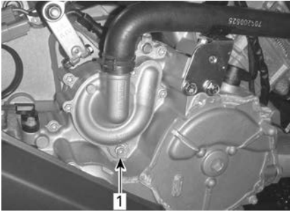
1. Jäähdytysnesteen tyhjennystulppa
