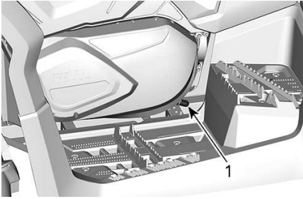
1. Depósito de drenaje de la CVT
