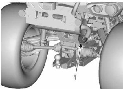
1. Conector del remolque
