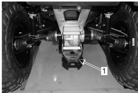
1. Hinterer Abschlepphaken
