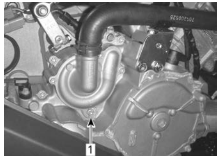
1. Kühlmittelablassschraube
