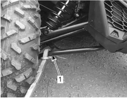
1. Etujousituksen alatukivarsi
