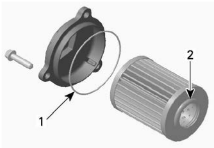
ETUMASKIN KANSI
