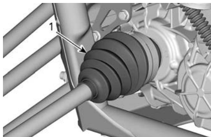
车辆后部（为方便观察已拆下部件）
