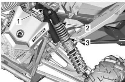
典型示例 - 不带回弹阻尼 - 前悬架
