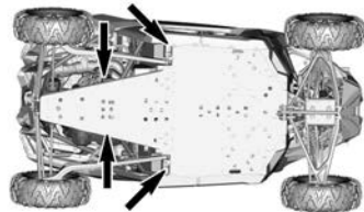
POSITIONS DES CHANDELLES - ARRIÈRE DU VÉHICULE
