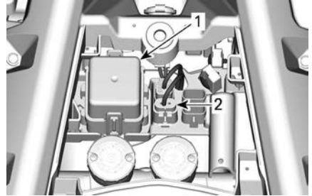
1. Boîte à fusibles avant 2. Fusible DPS
