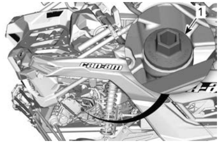
1. Пробка для проверки уровня масла коробки передач.
