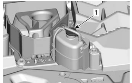
1. Герметизирующая крышка
