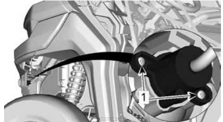
RIKTINGSVISARENS LAMPFATTNING
