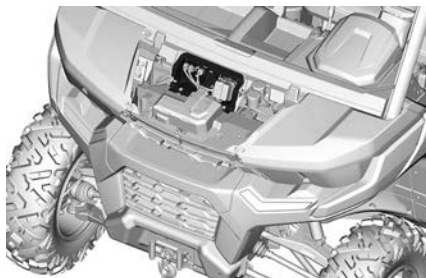
SÄKRINGSBOXENS STÖD
