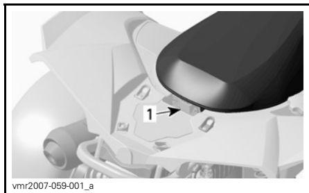
1. Grendel achteraan
