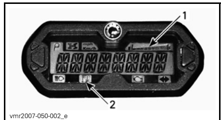
1. Brandstofpeilaanduiding 2. Verklikkerlichtje te laag brandstofpeil
