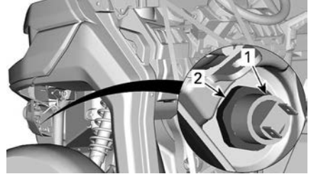
1. Feux de position 2. Écrou de retenue
