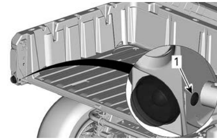
1. Linssin kiinnitysruuvi
