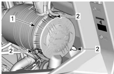
1. Крышка корпуса воздушного фильтра 2. Защелки
