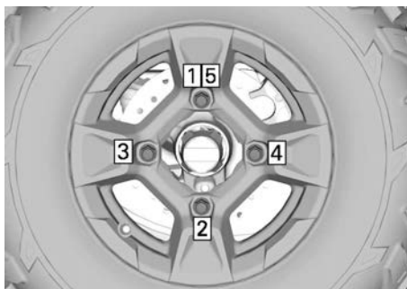
ПОРЯДОК ЗАТЯЖКИ
