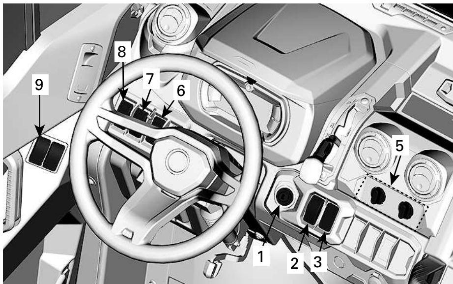
TYPIQUE - MODÈLE CAB AVEC CHAUFFAGE (PHOTO)
