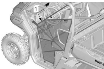
1. Filets latéraux
