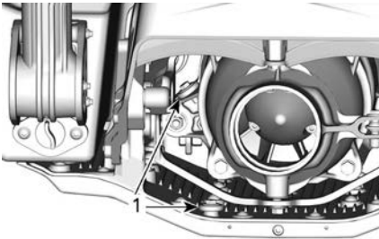
1. Anodes sacrificielles
