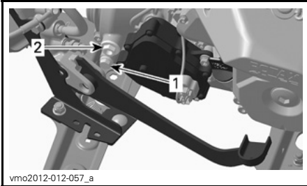
TÍPICO - MOTOR 1000
