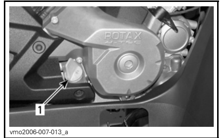
TÍPICO - LATERAL DERECHO DEL MOTOR
