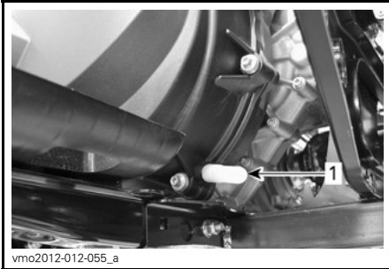
1. Depósito de drenaje de la CVT
