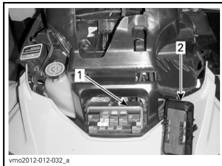
1. Meterhouder
