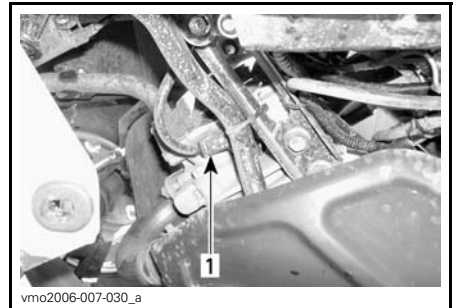
VASEN PUOLI — ETUSYLINTERI 1. Sytytystulppa
