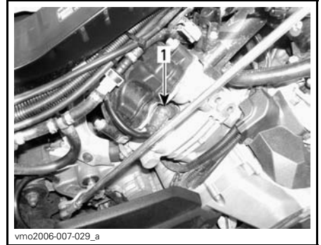
OIKEA PUOLI — TAKASYLINTERI 1. Sytytystulppa
