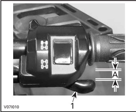
1. Kaasuvipu A. 3 mm - 6 mm
